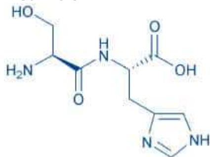
H-Ser-His-OH
