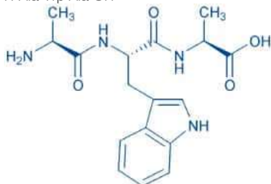
H-Ala-Trp-Ala-OH
