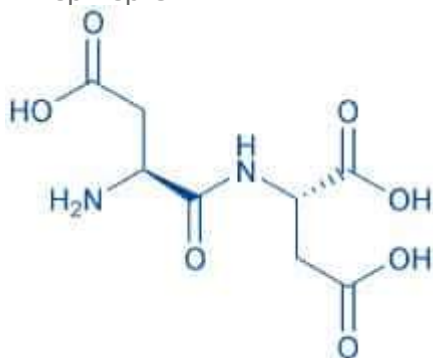
H-Asp-Asp-OH
