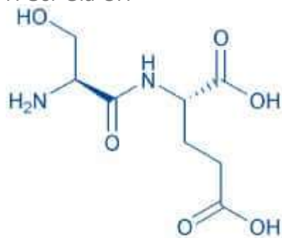
H-Ser-Glu-OH
