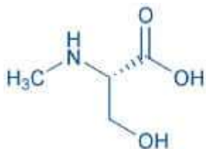
N-Me-Ser-OH
