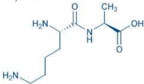
H-Lys-Ala-OH
