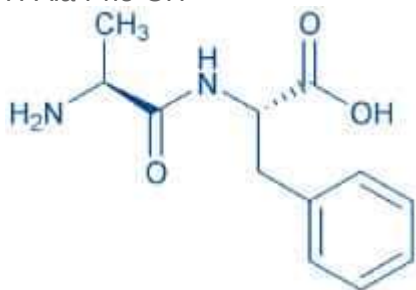
H-Ala-Phe-OH
